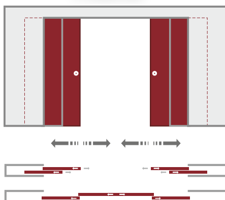
UȘI TELESCOPICE - INTERIOR PERETE 4 CANATURI
