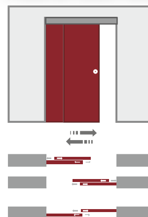
UȘI GLISANTE ÎNTRE PEREȚI - 2 CANATURI (DUBLU SENȘ)
